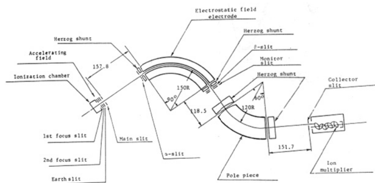
Obrázek 8. Schema přístroje JEOL JMS-D100, používaného Dr Hanušem of 70 let pro objasňování struktury organických a bioorganických látek
