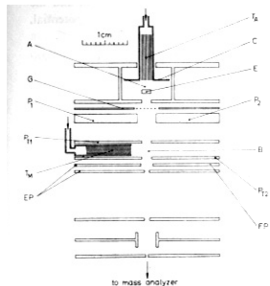
Obrázek 11. Iontový zdroj s molekulovými paprsky pro výzkum iontových produktů Penningovy ionizace
