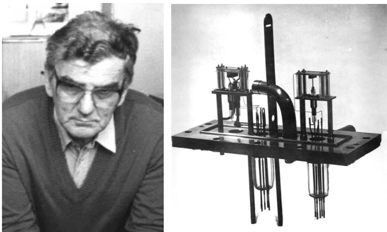
Obrázek 6. Dr. Zdeněk Dolejšek a výsledek jeho diplomové práce – malý hmotnostní spektrometr Dempsterova typu
