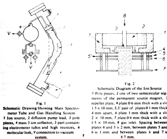
Obrázek 7: Schema přístrojů pro přesnou analýzu malých množství deuteria ve vodíku, postavených v ÚFCH ČSAV počátkem šedesátých let.
