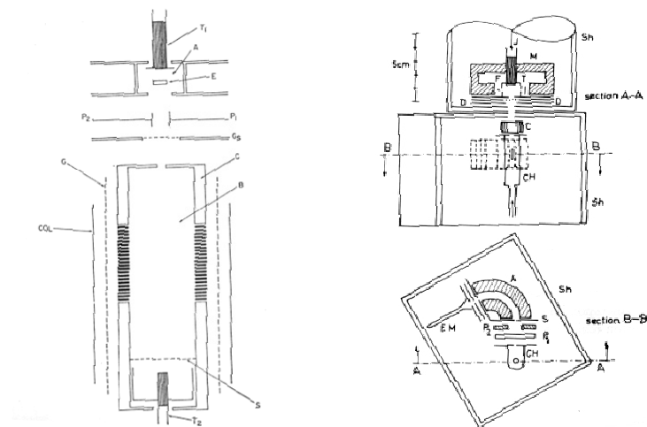
Obrázek 12. Čermákovy přístroje pro výzkum elektronové spektroskopie Penningovy ionizace (PIES): Lozierova trubice (vlevo) deflekční analyzátor energie elektronů (vpravo).
