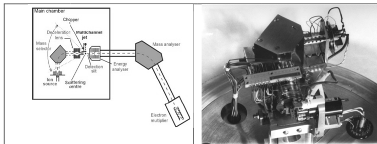
Obrázek 15a: Pražský přístroj EVA II pro výzkum dynamiky chemických reakcí iontů s molekulami, schema a pohled na vnitřní uspořádání zdrojů paprsků
