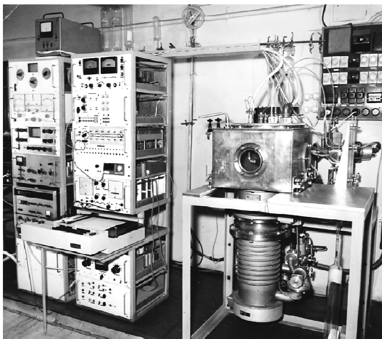
Obrázek 15b: Celý přístroj EVA II v r. 1973
