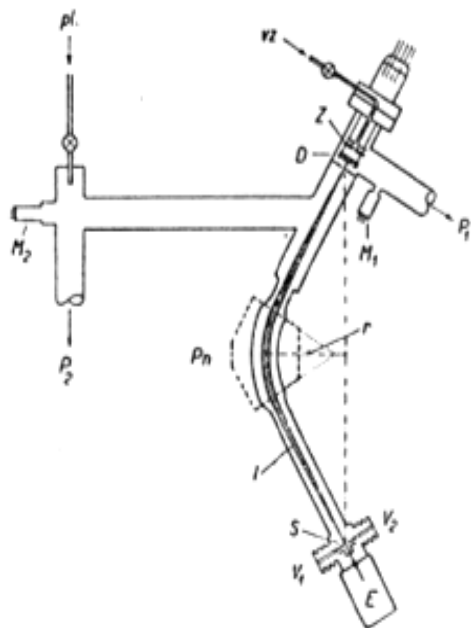
Obr. 1. Schéma trubice hmotového spektrometru.
