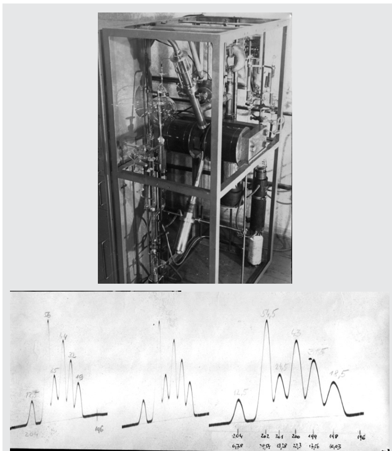
Obrázek 1: První hmotnostní spektrometr v ČSR a záznam prvního spektra rtuti (prosinec 1953)
