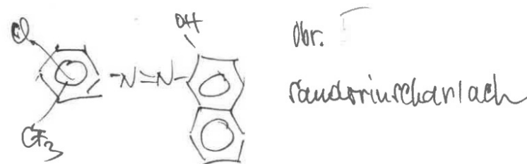
Obrázek 6: Strukturní vzorec Sandorinscharlach.
