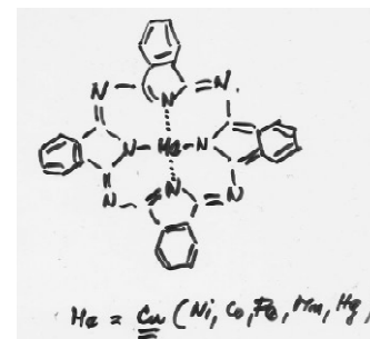
Obrázek 11: Barvivo ftalocyaninové modři
