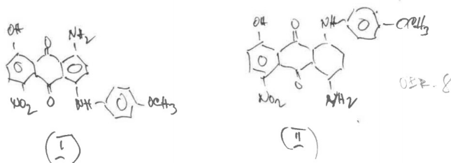
Obrázek 9: Vzorec I a vzorec II
