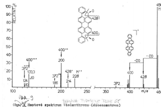
Obrázek 10: Spektrum barviva Pigment Blue 65
